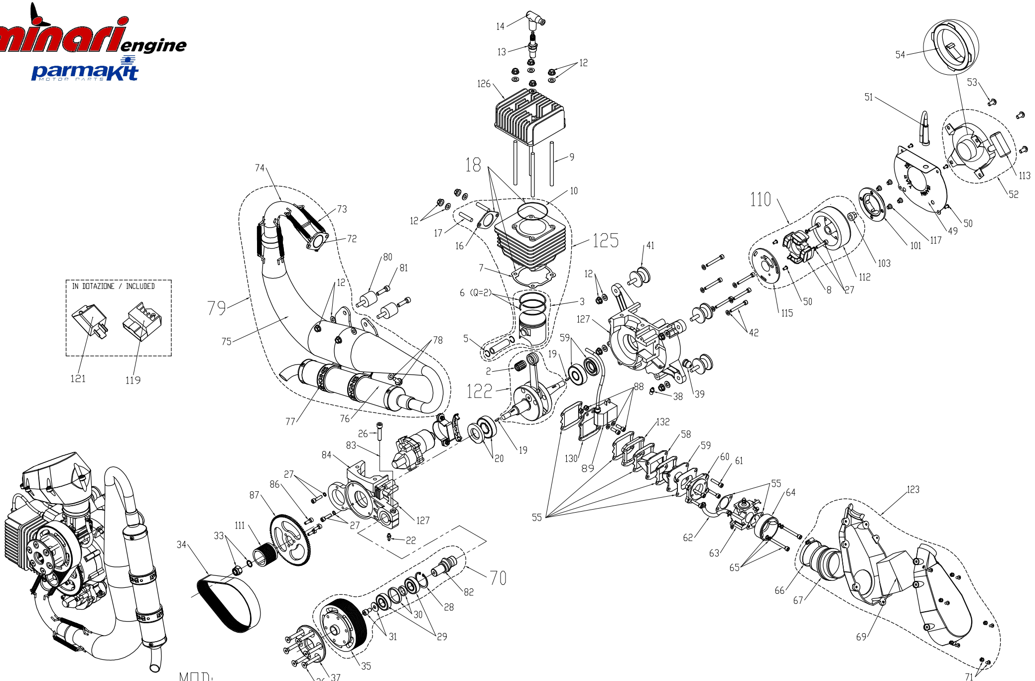
MOD: -F1-ME9C-CL CORSA LUNGA 200cc Motore a 90°, avviamento manuale + elettrico con carica / 90° engine, manual + electric starter with charger
