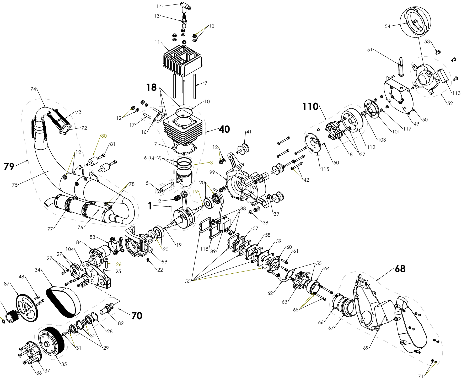
MOD: -F1-ME9C Motore a 90°, avviamento manuale + elettrico con carica batteria / 90° engine, manual + electric starter with charge battery
